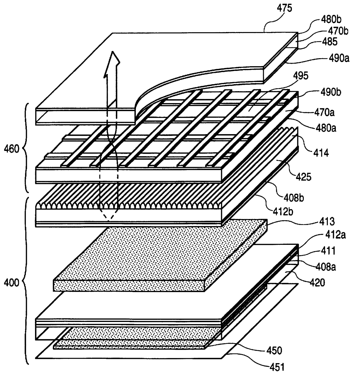
FIG. 4B
